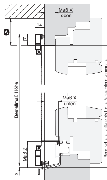
Vertikalschnitt
