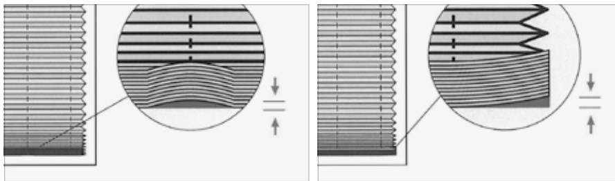
WELLIGKEIT IM BEREICH DES UNTERPROFILS Der zulässige Toleranzbereich beträgt 3 mm.
