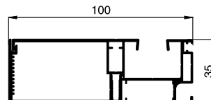
Führungsschiene bei Variante ER2/30
