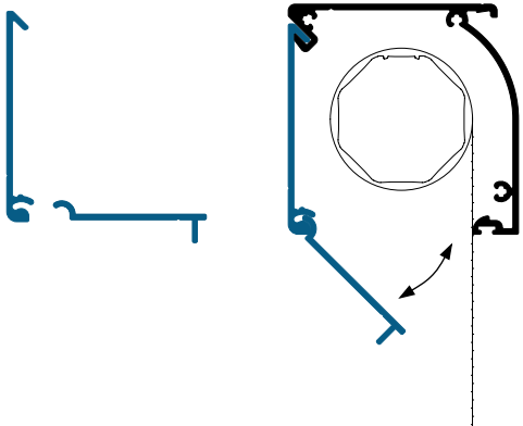
2-teilige Kastenblende
