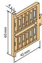
Distanzplatte bei Glastiefen unter 20 mm
