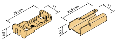
Montageset für F425 4 Schnurspanner Basis, 4 Deckel Schnurspanner, 4 Schrauben
