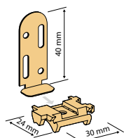
Träger Verbundfenster, zweiteilig Montageplatte mit Tragplatte
