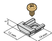
Basisteil für Spannschuh mit Schraube à 4
