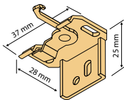
Wand-, Deckenträger mit Schnellspannung im Set inkl. Befestigung
