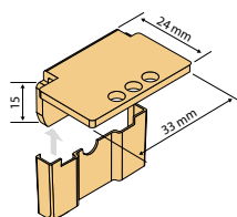
Wandwinkel mit Abdeckkappe für Spannschuh à 2 im Set inkl. Befestigung
