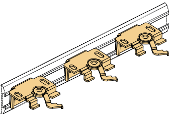
3er Zubehörset Klebprofil Wand-, Deckenträger
