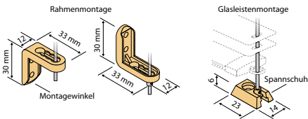
Universalset Kunststoff Standard für Pendelsicherung 2 Stk. Montagewinkel. 2 Stk. Spannschuh 2 Stk. Nippel, 4 Stk. Schrauben
