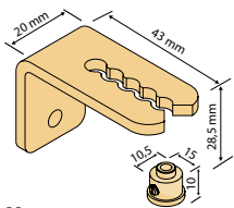
Montageset Spannwinkel und Stellring für Seilführung Inkl. Befestigungsmaterial 2 Stk. im Set
