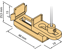
Klemmträger „Stelling“ für Pendelsicherung Klemmbereich 5 - 26 mm Abzug von Anlagenhöhe 15 mm
