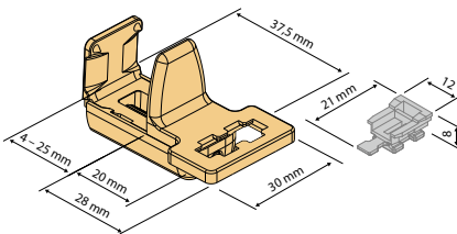
Klemmträger mit Dichtpad 2 Stück im Set Klemmbereich 4 - 25 mm
