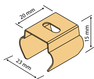
Deckenträger für Verbundfenster
