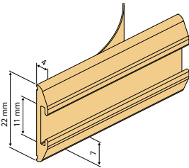
Klebprofil
