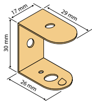
U-Träger
