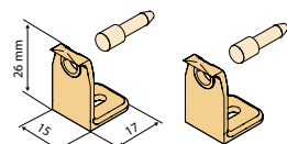
Unterprofilhalter Set 2 Unterprofilhalter, 2 Haltestifte, 2 Schrauben
