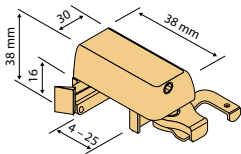
Klemmträger mit Schnellspannung und Dichtpad Klemmbereich 4 - 25 mm
