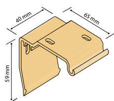
Wand-/Deckenträger inkl. Befestigung à 1 im Set
