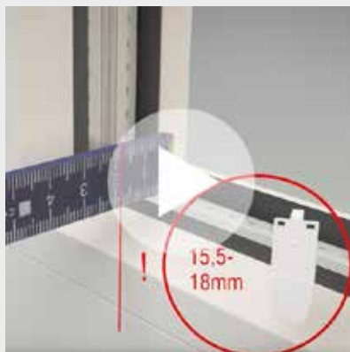
erfal VS2 Plisses mit Klemmträger Slim - Aufmaß bei schrägen Fensterfalz
