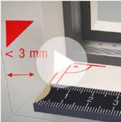
erfal VSC2 | ESC 2 Plissees – Aufmaß bei geraden Fensterfalz
