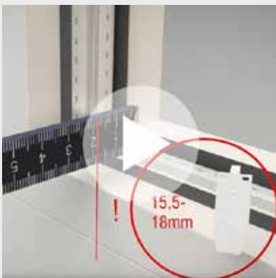
erfal VS2 Plisses mit Klemmträger Slim – Aufmaß bei geraden Fensterfalz
