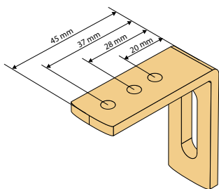
Wandwinkel 50 mm
