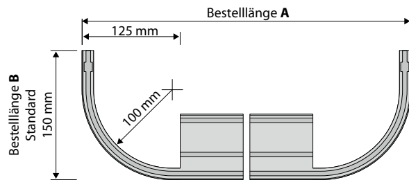
Retourenbiegung 4425/4430
