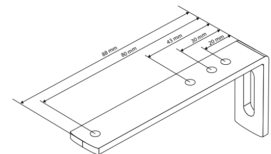
Wandwinkel 90 mm
