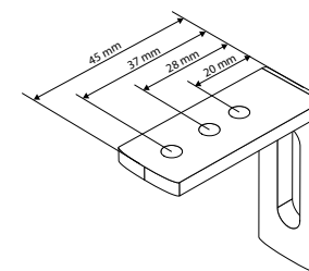
Wandwinkel 50 mm
