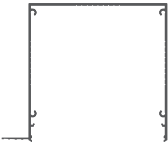
S-BOX 130 × 130 - NS (Flansch einseitig)
