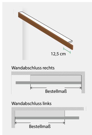
WANDANSCHLUSS EINSEITIG
