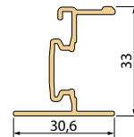
Seitenführungs-schiene
