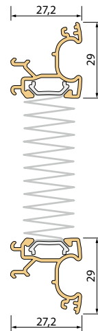
Seitenführungs-schiene
