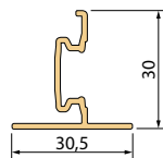
Seitliche Abdeckschiene
