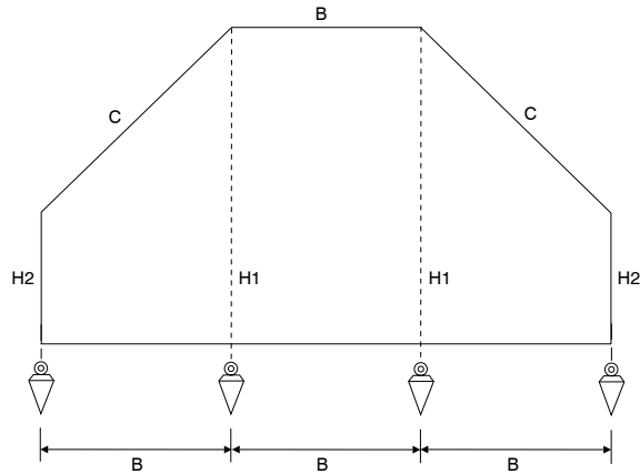
Rechte kozijnvleugel
