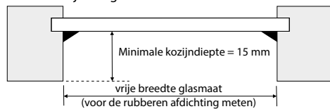
Schuine kozijnvleugel
