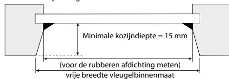
Schuine kozijnvleugel
