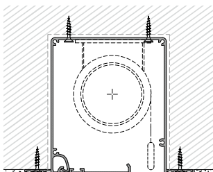
Installatievoorbeeld met een S-BOX 110 x 130 R
