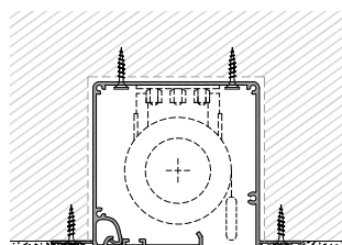
Installatievoorbeeld met een S-BOX 100x100 R
