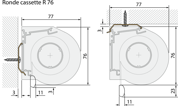
Ronde cassette R 76
