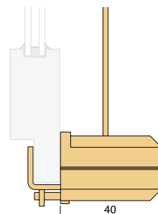
Klemsteunmontage op kozijn
