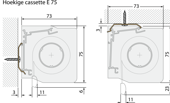
Hoekige cassette E 75
