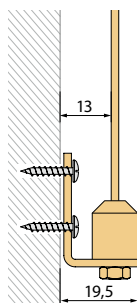
Wandmontage met hoeksteun
